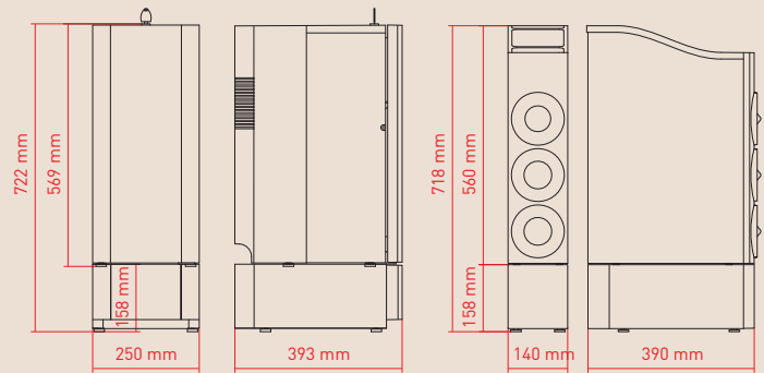
Seitliche Kühleinheit mit Sockel
